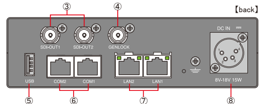
【front】① 電源スイッチ ② 操作コンソール 【back】③ SDI出力 ④ GENLOCK ⑤ USBポート ⑥ シリアルポート ⑦ LANポート ⑧ 電源コネクタ
